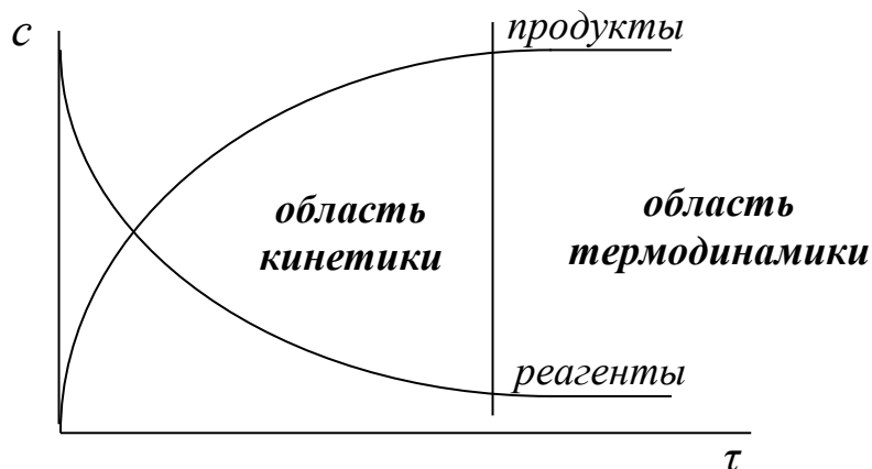
Рис. 3. Зависимость концентрации веществ ( c ) от времени ( \tau ) для обратимой химической реакции
